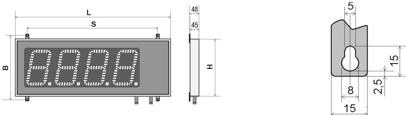
Rys.2.2.1. Widok wymiarowy wyświetlaczy LDN-x/100, LDN-x/150, LDN-x/227 Rys.2.2.2. Widok wymiarowy uchwyty
