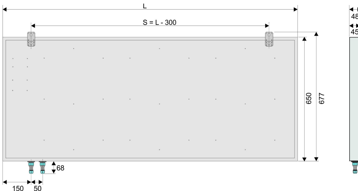
Rys.2.2.3. Widok wymiarowy wyświetlacza LDN-x/450
