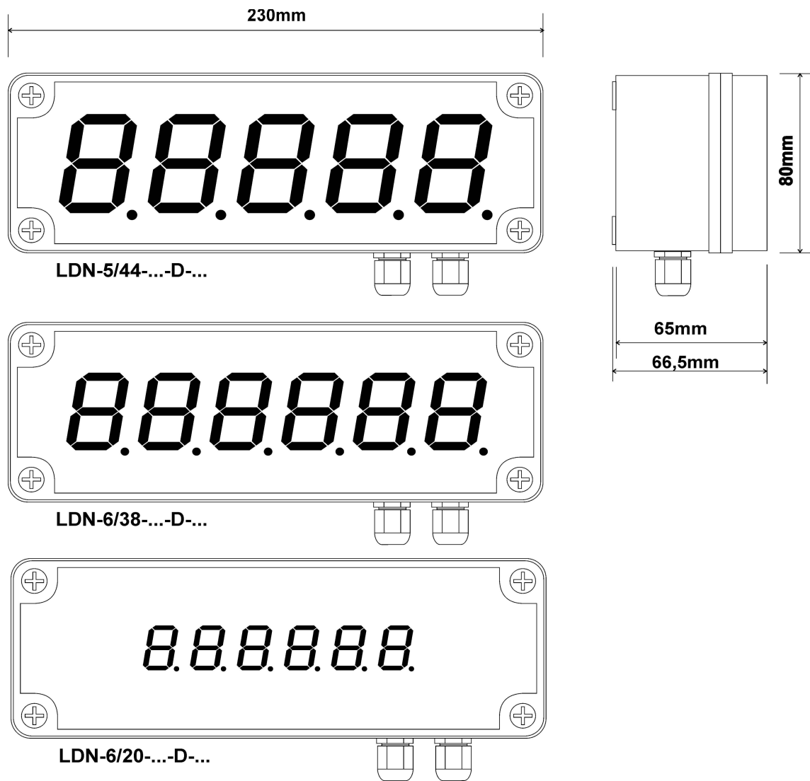
Rys. 2. Widok i wymiary wyświetlaczy LDN-...D-SBCD
