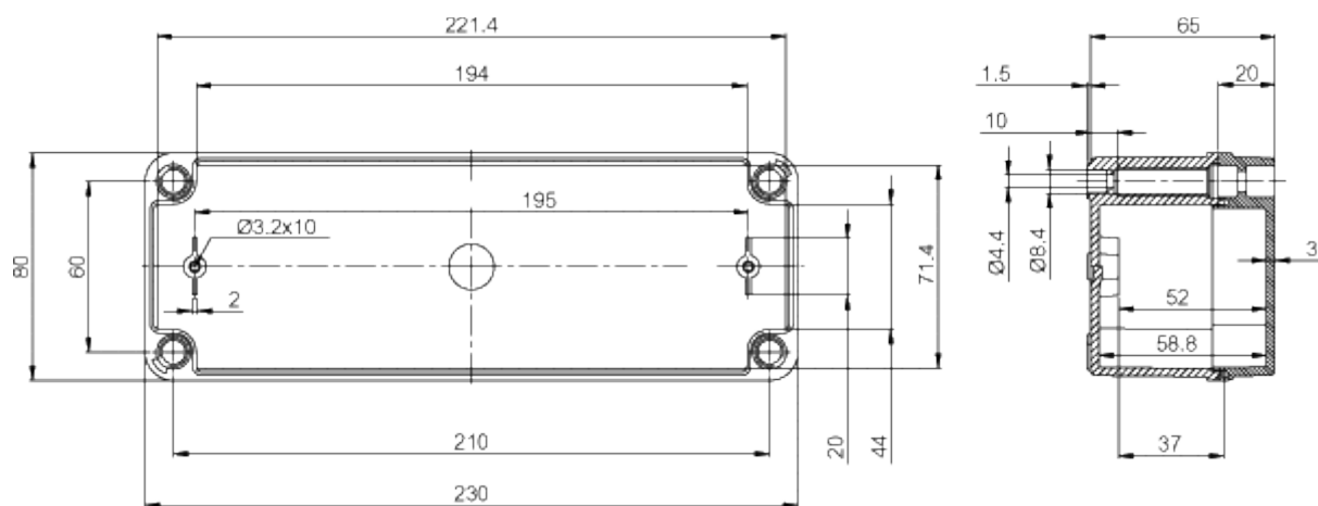
Rys. 3. Wymiary wyświetlaczy LDN-...D-
