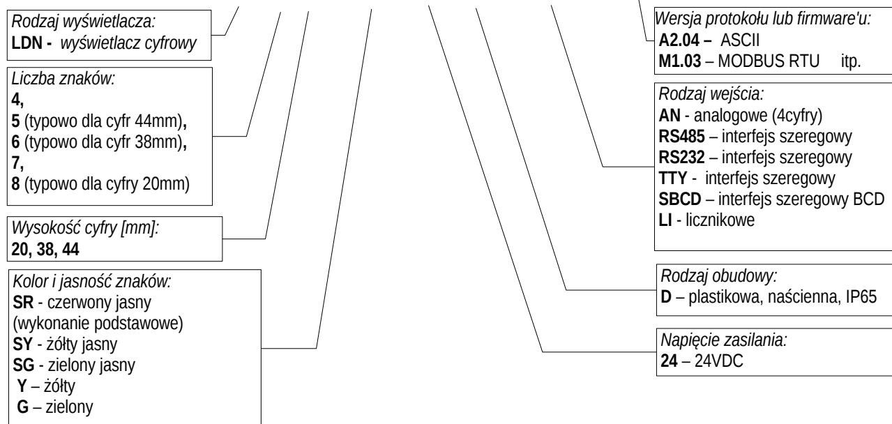
Rys. 1. Sposób oznaczenia wyświetlaczy tablicowych LDN-...-D-...
