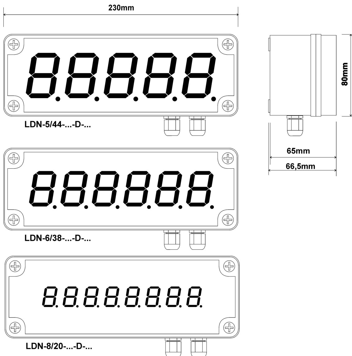
Rys. 2. Widok i wymiary wyświetlaczy.
