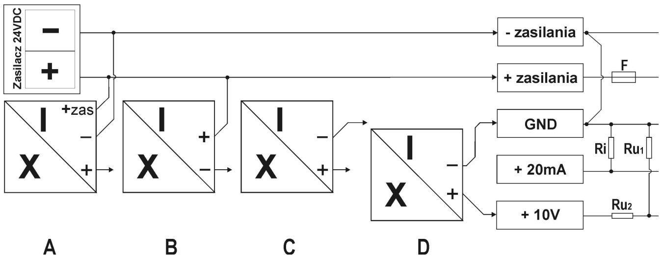
Rys.1. Przykładowe schematy połączeń przetworników pomiarowych.
