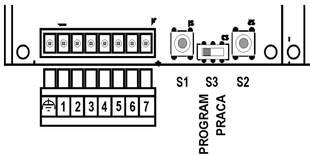
Rys.2. Widok złącza i przycisków programujących - moduł kontrolera
