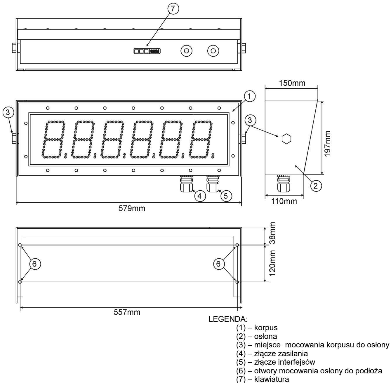
Rys.2. Widok i wymiary wyświetlacza – LDN-(4)(5)(6)/100D-... lub LDN-(4)(5)/100-...
