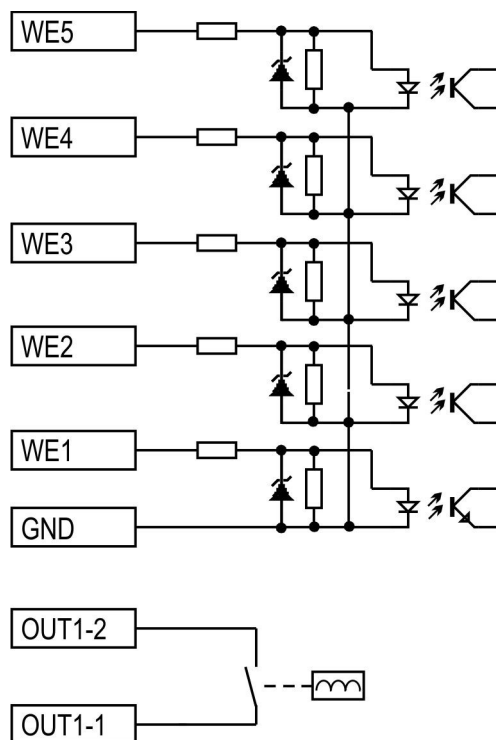
Rys. 4. Wejścia/wyjścia – schemat uproszczony
