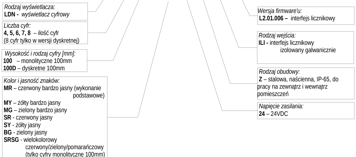
Rys.1. Sposób oznaczenia wyświetlaczy naściennych LDN-x/100D-...-Z-ILI
