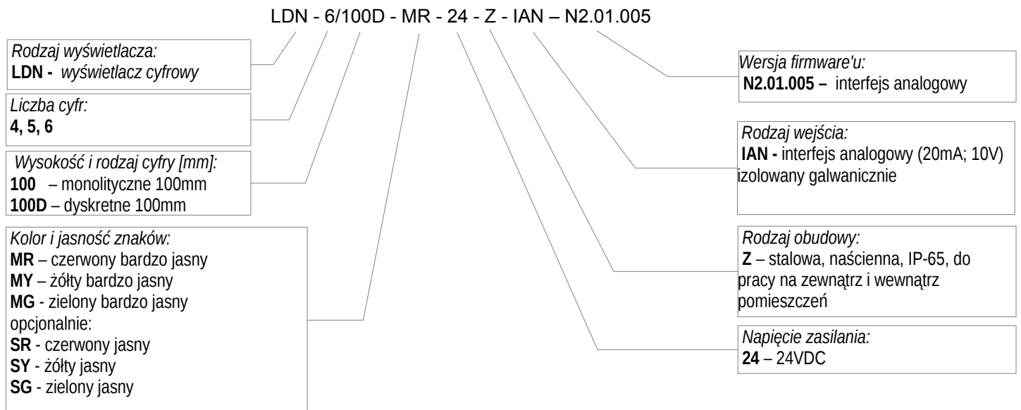
Rys.1.5.1. Sposób oznaczenia wyświetlaczy naściennych LDN-x/100D-...-Z-IAN
