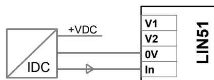
Podłączenie przetwornika prądowego 3 przewodowego.
