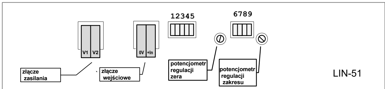
Widok płyty tylnej przyrządu.
