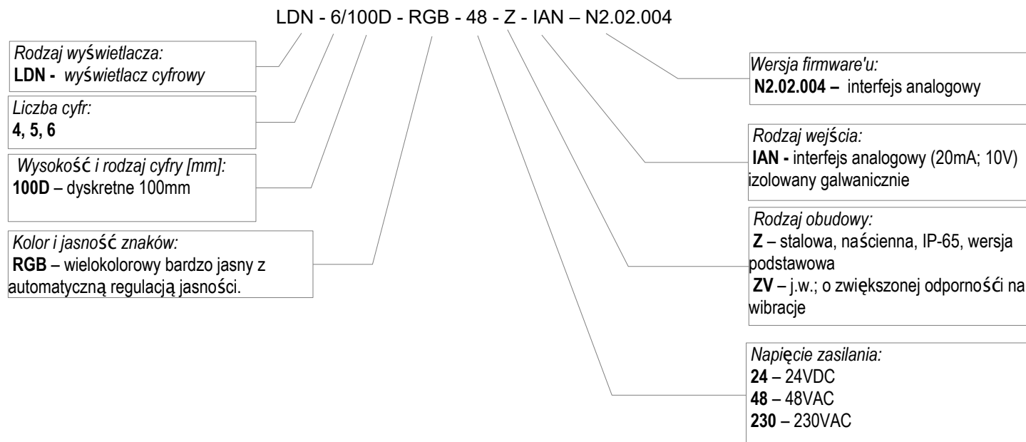
Rys.1.5.1. Sposób oznaczenia wyświetlaczy naściennych LDN-x/100D-RGB-...-Z(V)-IAN
