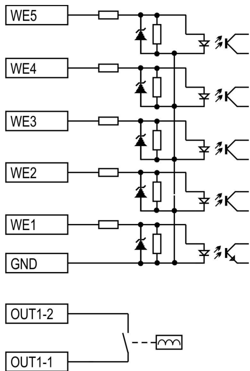
Rys. 2.3.1. Wejścia/wyjścia – schemat uproszczony
