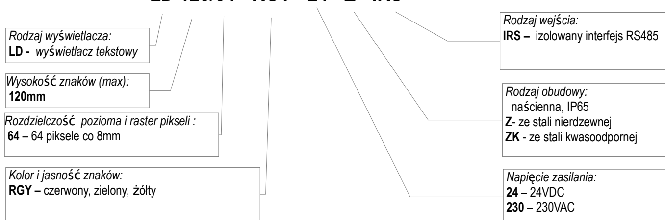
Rys.1 Sposób oznaczania wyświetlaczy LD120-...
