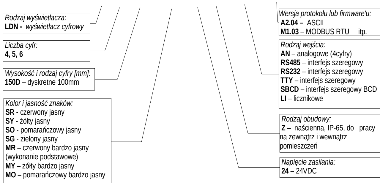
Rys. 1. Sposób oznaczenia wyświetlaczy naściennych LDN-x/150D-...-Z-...
