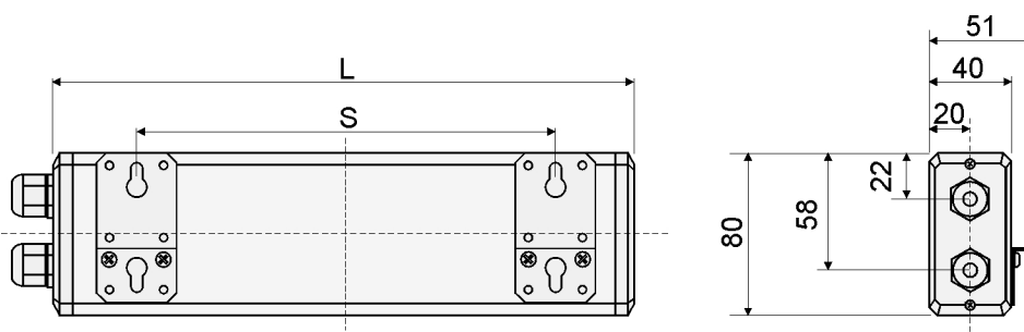
Rys. 5. Wymiary obudów stosowanych do cyfr o wysokości 44mm (LDN-x/44-...).
