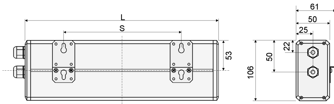
Rys. 5. Wymiary obudów stosowanych do cyfr o wysokości 57mm (LDN-x/57-...).
