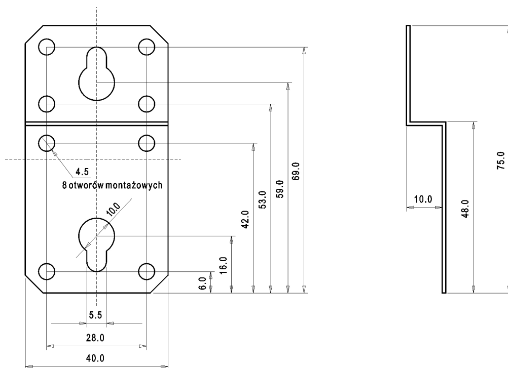
Rys. 6. Wymiary uchwyty ściennego
