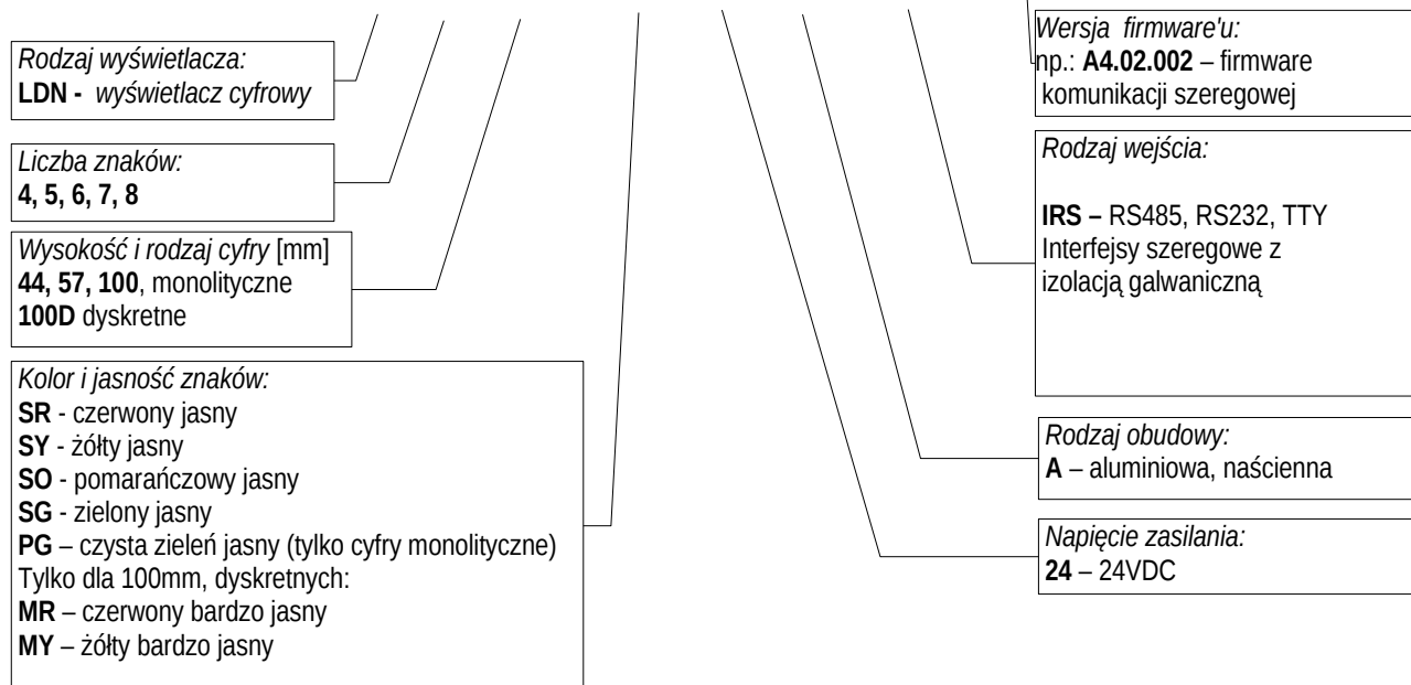
Rys. 1. Sposób oznaczenia wyświetlaczy naściennych LDN-...-A-IRS-...
