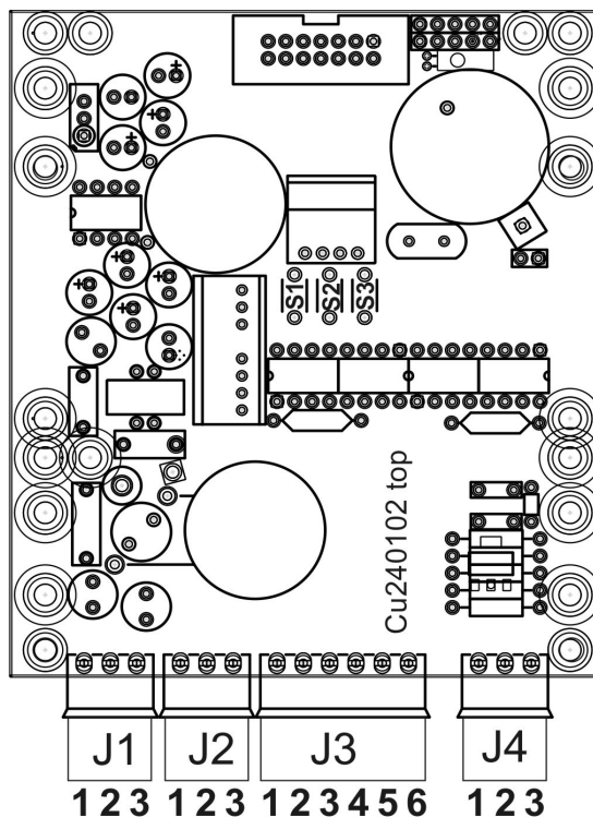
Rys.7 Widok płytki kontrolera. Położenie i numeracja złącz i przycisków.
