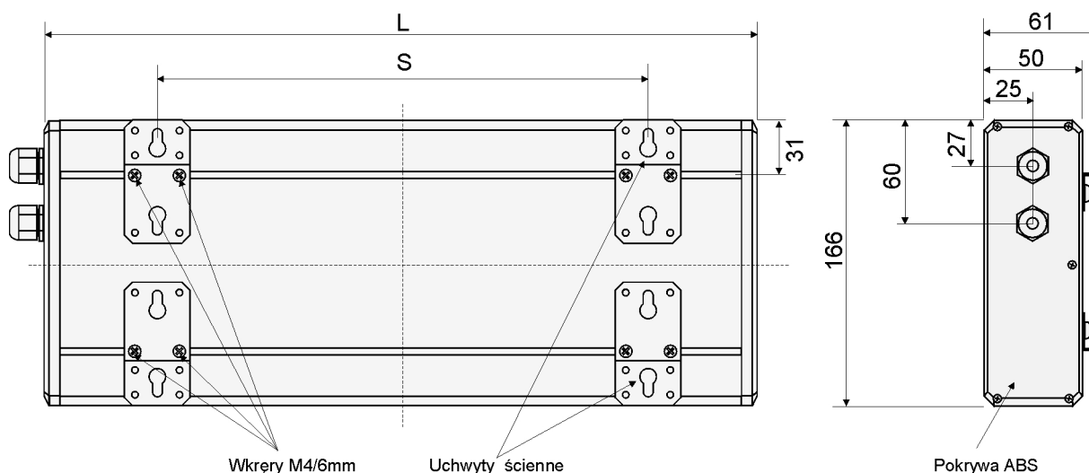
Rys. 4. Opis i wymiary obudów stosowanych do cyfr o wysokości 100 mm (LDN-x/100...).
