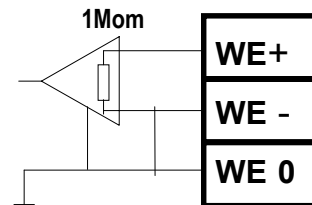
Wejście pomiarowe napięciowe
