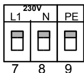
Opis złącza zasilania w wersji 230V.
