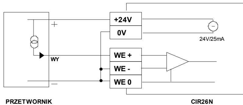
Podłączenie trójprzewodowe
