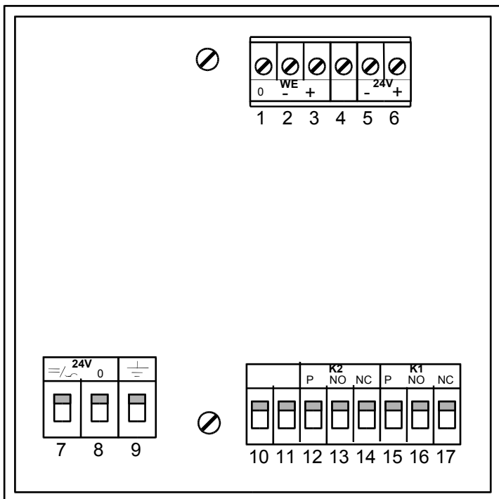
Płyta tylna miernika w wersji 2 progowej
