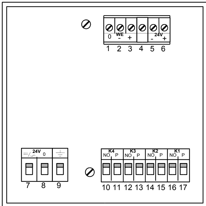
Płyta tylna miernika w wersji 4 progowej.
