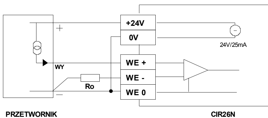
Podłączenie czteroprzewodowe
