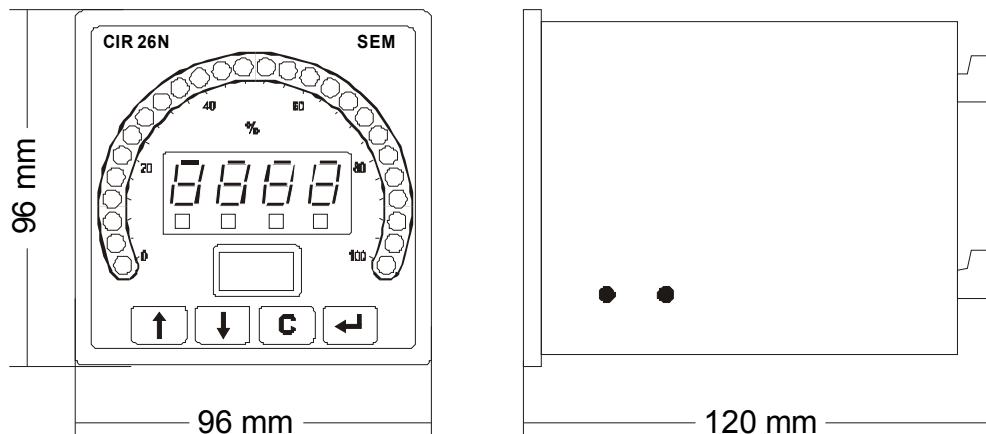
Wymiary przyrządu.
